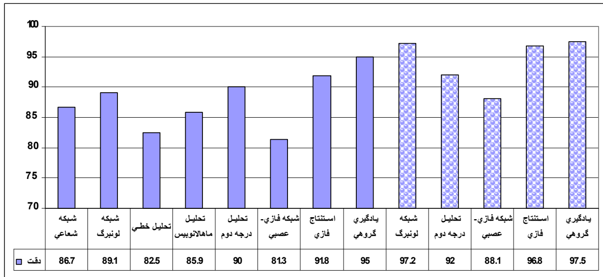
شکل ۵- مقایسه نتایج طبقه بندی کنندگان مختلف
