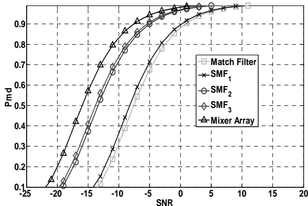
شکل ۹- احتمال آشکار سازی رادار به صورت تابعی از SNR برای F_d = 4 \text{ KHz} و P_{fa} = 10^{-6}
