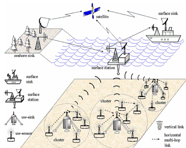
شکل ۱- نمونه‌ای از یک شبکه زیر دریا (اقتباس از [۱])
