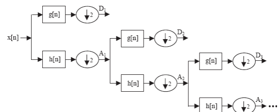
شکل ۳- فرآیند تجزیه چندمرحله‌ای موجک از سیگنال x[n]
